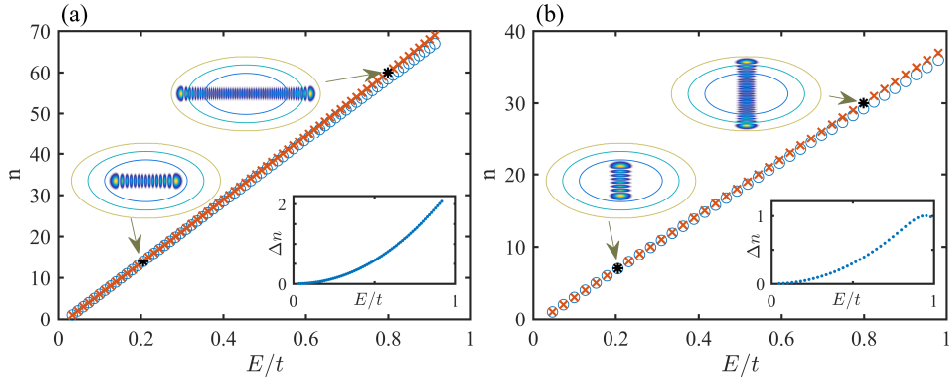
图 4 小扰动下二维谐振子势中的 Bouncing ball 量子态的轨道方向量子数 n 对能量的依赖图。叉号为根据波函数数出来的波长数减 1，圆圈为根据半经典公式得到的 n 。(a) 为横向 bouncing ball 态，(b) 为纵向 bouncing ball 态。小图 \Delta n 为根据波函数数出来的结果和根据本征能量计算出来的结果的差。
