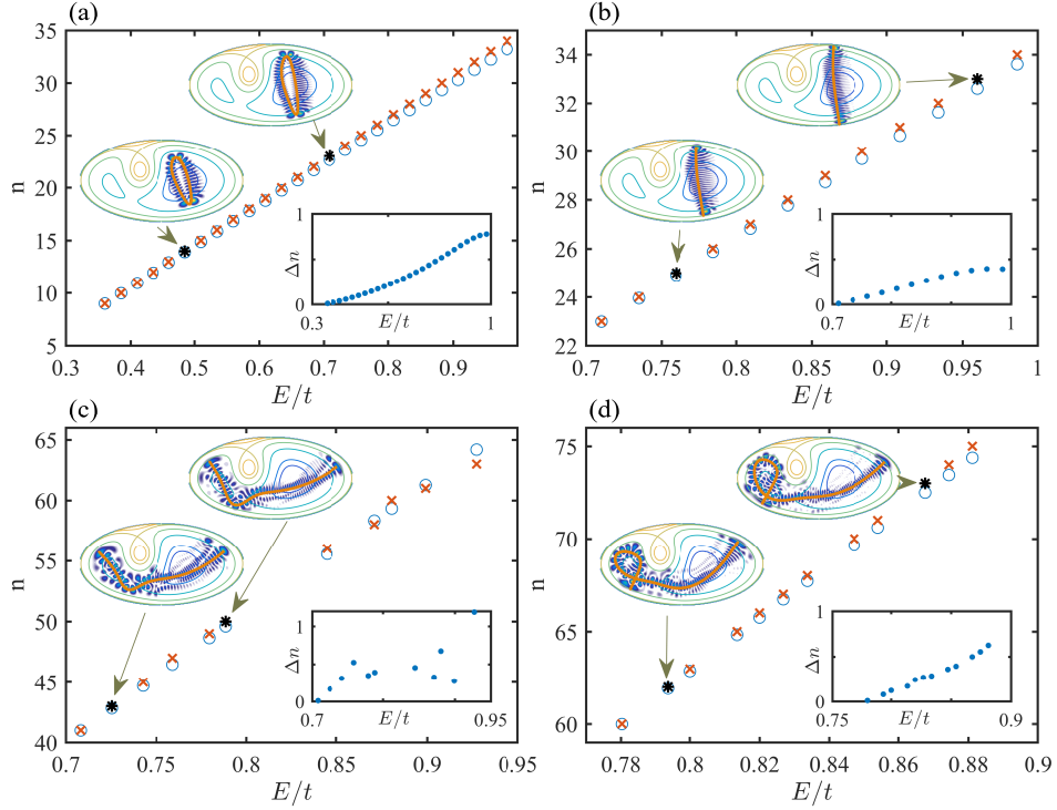
图 8 沿轨道方向量子数 n 与能量的依赖关系。叉号为根据波函数数出来的波长数减 1，圆圈为根据半经典公式得到的 n 。这里所有态的横截量子数 m 均为 0。(a-d) 分别对应第三类(C3)、第四类(C4)、第五类(C5)、第六类(C6)轨道，对应的 E_o 分别为 0.0220t , 0.0013t , 0.0280t , 和 0.0193t 。图中小图展示了一些标准的疤痕态及其对应的经典轨道，以及两种 n 的差值。C3 只在能量为 0.35t 时 C2 失稳后才出现。C4 为 C2 的另外一支不稳定轨道，只在能量超过 0.95t 后才稳定。C5 和 C6 是连接两个势谷的轨道，只在较高能级时出现。
