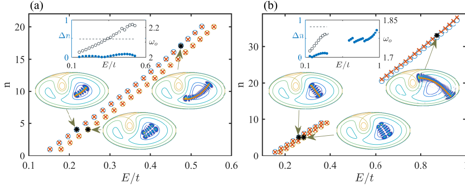
图 7 沿轨道方向量子数 n 与能量的依赖关系。叉号为根据波函数数出来的波长数减 1，圆图为根据半经典公式得到的 n 。(a) 第一类 bouncing ball 轨道 (C1); (b) 第二类 bouncing ball 轨道 (C2)。每个图中横截量子数 m=0 为上面那组点， m=1 的为下面那组点。对于 C2 轨道，只有能量较低的时候有 m=1 的量子态，能量较高时在计算中没有发现 m=1 的态。图中小图展示了一些标准的疤痕态及其对应的经典轨道，两种 n 的差值（蓝色实心圆，左侧坐标）以及由 E_{n,1} - E_{n,0} 计算出的 \omega_o 值（黑色空心圆，右侧坐标），其中横虚线为拟合得到的 \omega_o 值 ( \omega_o L_o / \sqrt{2} a )，对应的 E_o = \hbar \omega_o / 2 分别为 0.0141t 和 0.0121t 。
