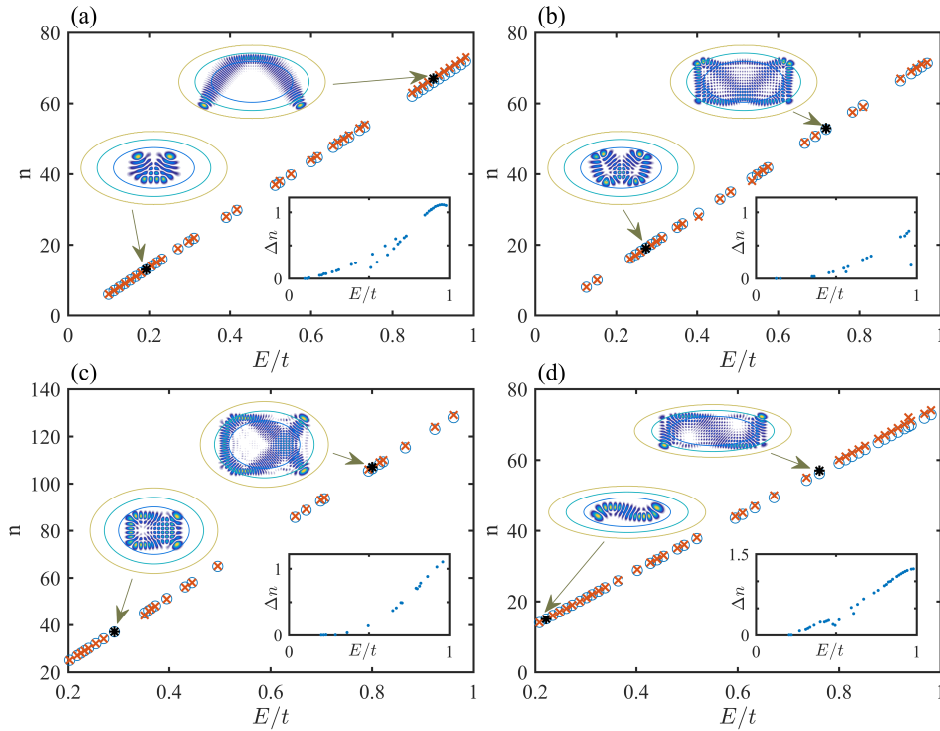
图 5 小扰动二维谐振子势场中 4 类李萨如态的量子化条件。叉号为根据波函数数出来的波长数减 1，圆圈为根据半经典公式得到的 n 。图中小图为根据波函数数出来的结果和根据本征能量计算出来的结果的差。
