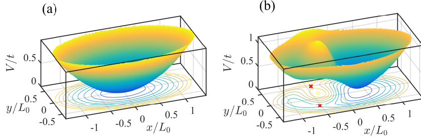
图 1 (a)二维谐振子势[公式(2)], 其中 L_0 是系统的特征尺度, \omega'_x L_0/\sqrt{2}a = 1 , \omega'_y = 2\omega'_x 。为了破坏对称性, 我们在 (x_\delta/L_0, y_\delta/L_0) = (-0.278, -0.226) 处加了一个 \delta(x - x_0, y - y_0) 函数势。(b)在势场(a)的基础上, 加入了一个高斯势场 V_G = U e^{-[(x-x_G)^2 + (y-y_G)^2]/(2\sigma^2)} , 其中 U = 1t , \sigma/L_0 = 0.2828 , (x_G/L_0, y_G/L_0) = (-0.3441, 0.1226) 。这样整个势场形成左右两个谷, 一个峰, 其中右侧谷底的位置为 (x_V/L_0, y_V/L_0) = (0.3574, -0.0179) , 对应的势能为 V_{\min} = 0.1053t 。两个势谷之间存在两个鞍点, 如叉号所标示的位置, 对应的势能分别为 0.591t 和 0.976t 。
