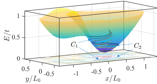
图 6 大扰动二维谐振子势场中的两类 bouncing ball 轨道以及它们在零能量面上的投影。纵轴对应的是每个轨道的能量值。为了便于辨认, 势函数及其等势线也一起画在了图上。第一组(C1)轨道对应着图 2 中在 p_{//} = 0 , \theta/2\pi \approx 0.1 和 0.6 处两个最显著的 KAM 岛的中心轨道, 第二组(C2)轨道对应着图 2(a) 中在 p_{//} = 0 , \theta/2\pi \approx 0.33 和 0.86 处两个 KAM 岛的中心轨道。
