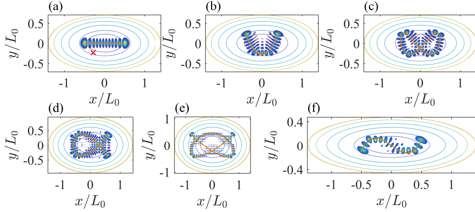
图 3 图 1(a)势场下粒子的本征态。图中所画为一些具有代表性的波函数的模方，凝聚在李萨如轨道上。x 和 y 方向的频率比为(a-c) 1:2, (d) 2:3, (e) 3:4, (f) 1:3。对所有情况， \omega_x L_0 / \sqrt{2}a = 1 ， x/L_0 的范围为 [-\sqrt{2}, \sqrt{2}]L_0 ，谐振子势在 y = 0 的边界上的值为 1\tau 。
